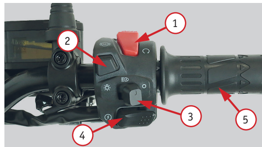
Фото 2.5. Правый комбинированный переключатель: 1 – кнопка включения/отключения питания; 2 – кнопка ABS, кнопка включения/выключения света; 3 – включить освещение; 4 – электростартер; 5 – ручка газа (акселератора)
