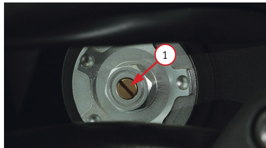
Фото 2.14. Регулировка демпфирования переднего и заднего амортизатора: регулирующий винт - 1
