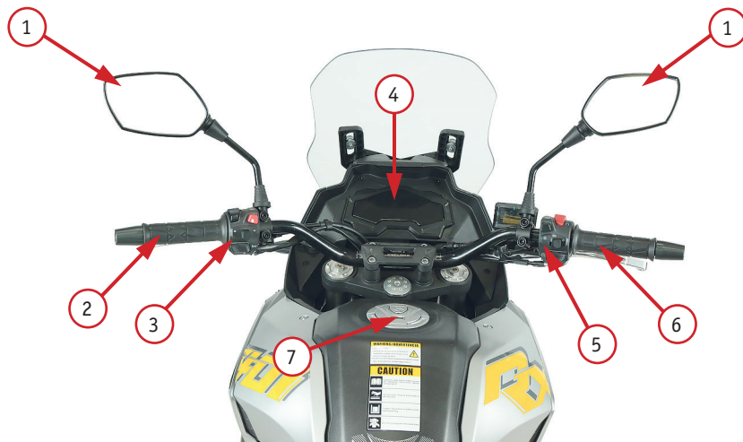
Фото 2.1. Вид руля и органов управления мотоцикла: 1 – зеркало заднего вида; 2 – левая рулевая рукоятка; 3 – левый комбинированный переключатель; 4 – приборная панель; 5 – правый комбинированный переключатель; 6 – рукоятка газа (акселератор); 7 – крышка топливного бака
