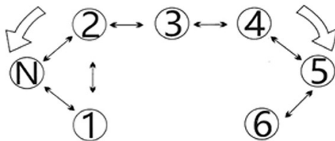
Рисунок 1. Схема переключения передач
