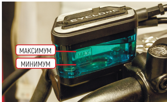
Фото 5.8.2. Бачок тормозной жидкости передних тормозов
