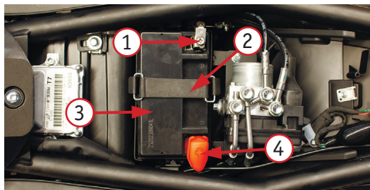
Фото 4. Аккумуляторный отсек: 1 – клемма «минус»; 2 – ремень крепления аккумуляторной батареи; 3 – аккумуляторная батарея (АКБ); 4 – колпачок клеммы «плюс»
