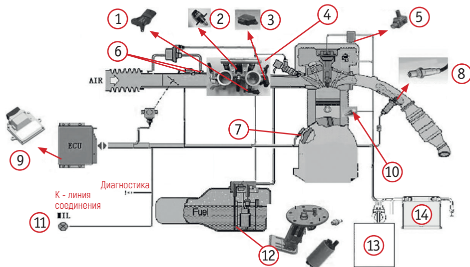
Схема 1. Схема системы EFI: 1 – датчик давления/температуры всасываемого воздуха; 2 – регулятор холостого хода; 3 – датчик положения дроссельной заслонки; 4 – топливный дроссель в сборе; 5 – катушка зажигания; 6 – корпус дроссельной заслонки; 7 – датчик положения коленчатого вала; 8 – датчик кислорода; 9 – электронный блок управления двигателем (ЭБУ); 10 – датчик температуры двигателя; 11 – лампа сигнализации о неисправности; 12 – топливный насос с кронштейном; 13 – насос топливный / клапан регулирования давления / фильтр тонкой очистки; 14 – аккумуляторная батарея (АКБ)
