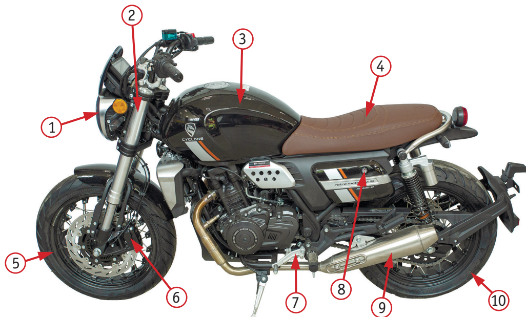
Фото 2.3. Вид слева: 1 – передняя фара; 2 – передний амортизатор; 3 – топливный бак; 4 – сиденье; 5 – переднее колесо; 6 – передний тормозной суппорт; 7 – рычаг переключения передач; 8 – замок сиденья; 9 – глушитель; 10 – заднее колесо
