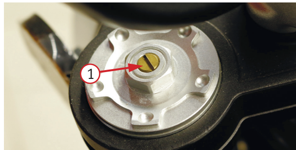
Фото 2.14. Регулировка демпфирования переднего амортизатора: регулировочный винт 1
