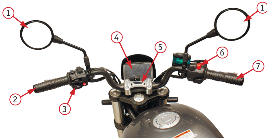
Фото 2.1. Вид руля и органов управления мотоцикла: 1 - зеркало заднего вида; 2 - левая рулевая рукоятка; 3 - левый комбинированный переключатель; 4 - приборная панель; 5 - замок зажигания (рядом с панелью); 6 - правый комбинированный переключатель; 7 - рукоятка газа (акселератор)
