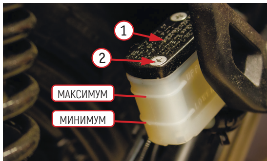
Фото 5.8.1. Бачок тормозной жидкости задних тормозов: 1 – крышка бачка; 2 – винты крепления крышки бачка
