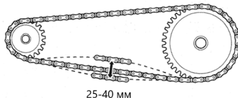
Рисунок 3. Натяжение цепи
