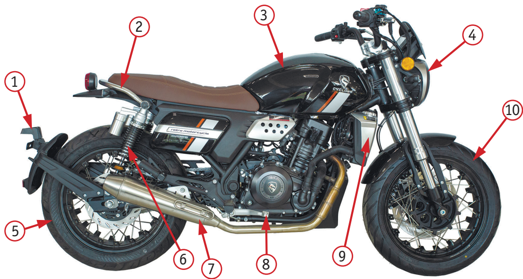
Фото 2.2. Вид справа: 1 - фонарь освещения номерного знака; 2 - пассажирский поручень; 3 – топливный бак; 4 – передняя фара; 5- заднее колесо; 6 - задний амортизатор; 7 - глушитель; 8 – рычаг заднего тормоза; 9 - радиатор; 10 - переднее колесо
