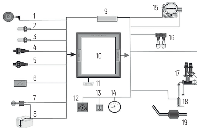
Схема 1. Схема системы EFI: 1 – датчик положения коленчатого вала; 2 – датчик кислорода L; 3 – датчик кислорода R; 4 – термодатчик двигателя; 5 – датчик температуры/давления всасываемого воздуха; 6 – выключатель нейтральной передачи; 7 – замок зажигания; 8 – аккумуляторная батарея; 9 – сигнализатор нештатного воздействия; 10 – модуль управления двигателем; 11 – разъем для диагностики неисправностей/последовательный интерфейс связи; 12 – индикатор неисправности; 13 – контрольная лампа повышенной температуры двигателя; 14 – сигнал скорости вращения двигателя; 15 – датчик положения дроссельной заслонки; 16 – катушка зажигания; 17 – WCPR регулятор давления топлива; 18 – топливный насос; 19 – каталитический нейтрализатор
