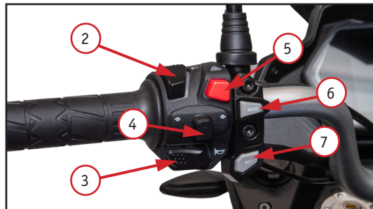
Фото 2.4. Левый комбинированный переключатель: 2 – кнопка переключения режима света фары (дальний свет/ближний свет); 3 – кнопка звукового сигнала; 4 – кнопка указателей поворота; 5 – кнопка включения аварийной сигнализации; 6 – кнопка «MODE»; 7 – кнопка «SET»
