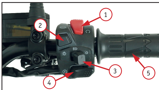
Фото 2.5. Правый комбинированный переключатель: 1 – кнопка включения/отключения питания; 2 – кнопка ABS; 3 – кнопка включения/выключения света фар; 4 – электростартер; 5 – ручка газа (акселератора)
