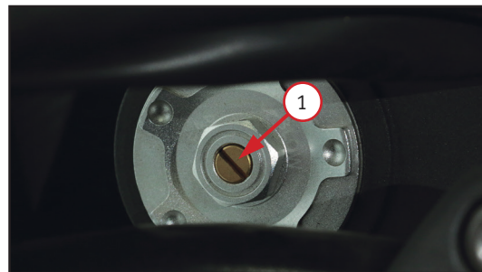
Фото 2.14. Регулировка демпфирования переднего и заднего амортизатора: регулируемый винт - 1
